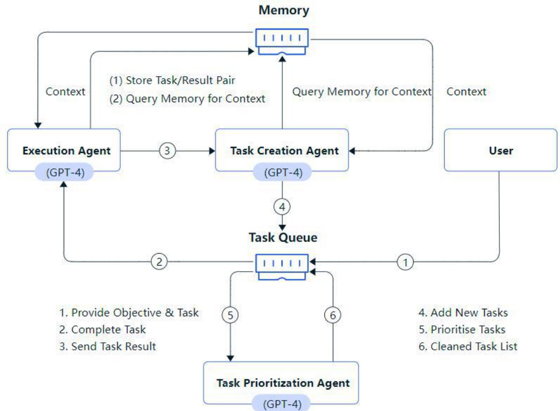
图 52: AutoGPT 的工作流程
